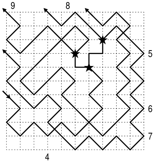
Finale 3 Teilchenzoo
