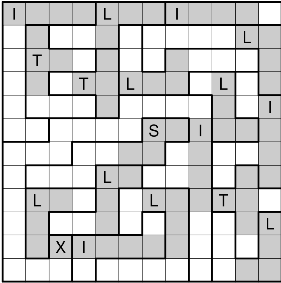
Finale 1 Zusatzschwarzfeld-LITS
