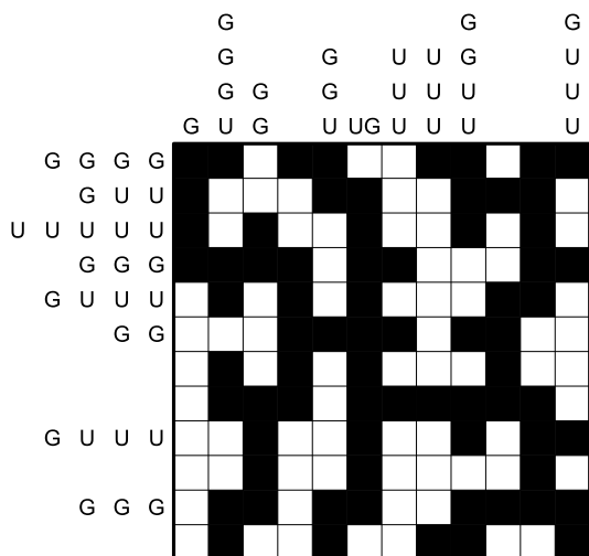
Finale 5 GU-Koralle
