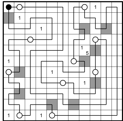
Finale 2 A 38
